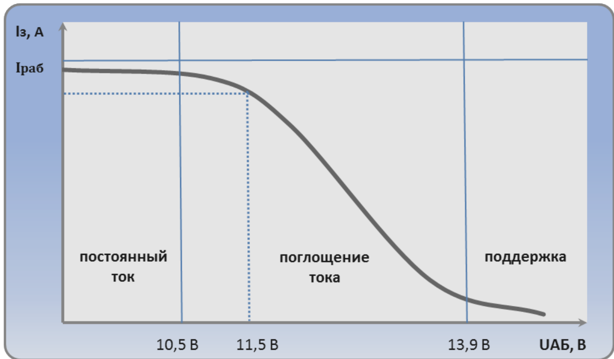
Мал.4. Графік роботи зарядного пристрою. Покращений заряд по Вубріджу (тристадійний режим заряду)
