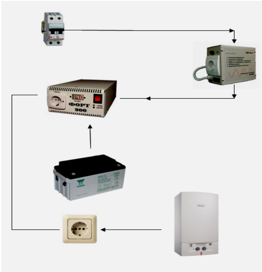
Рис.2. Приклад підключення інвертора ФОРТ з використанням стабілізатора
