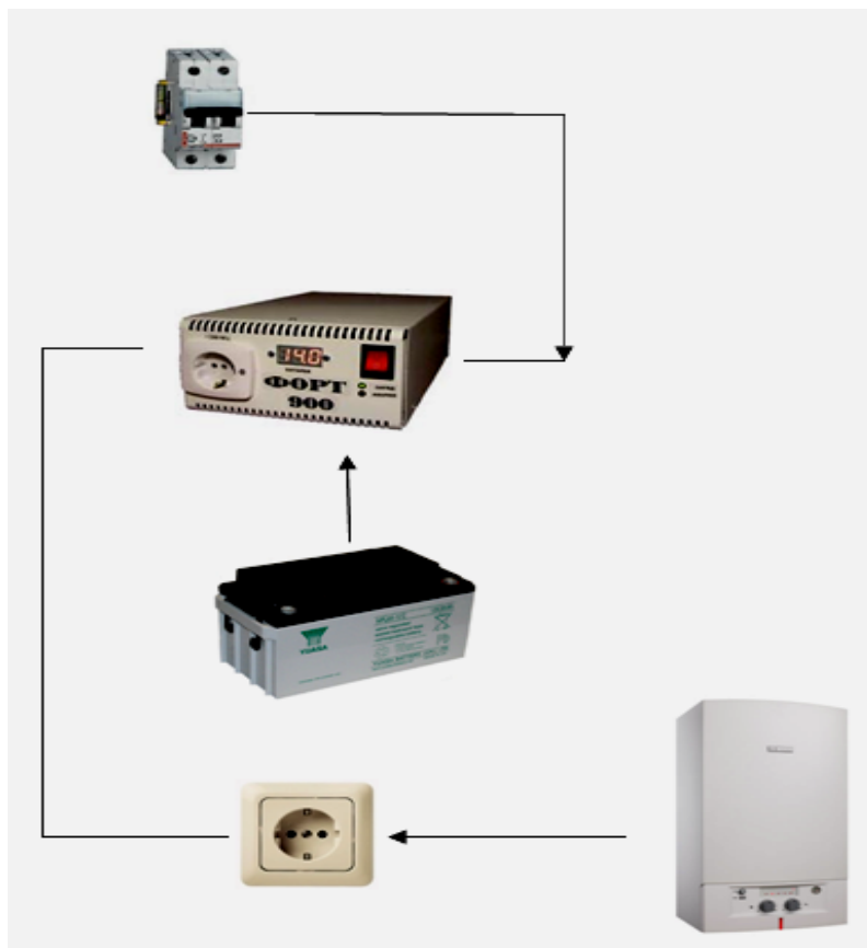
Рис.3. Приклад підключення інвертора ФОРТ без використання стабілізатора
